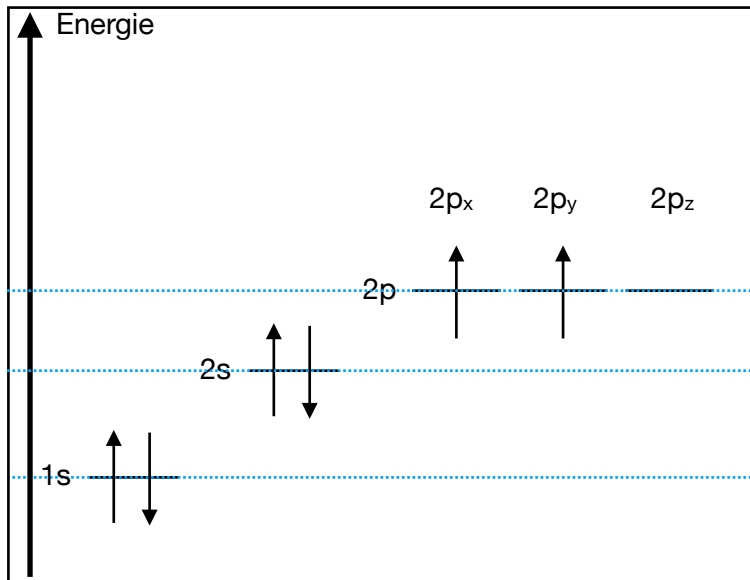
nichthybridisiertes C-Atom
