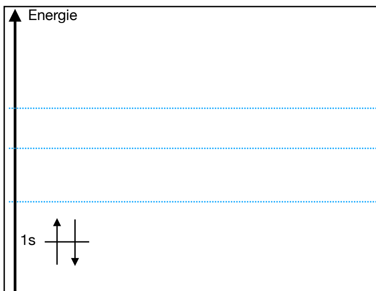
sp 2 -hybridisiertes C-Atom
