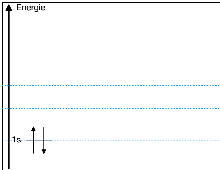
sp 3 -hybridisiertes C-Atom
